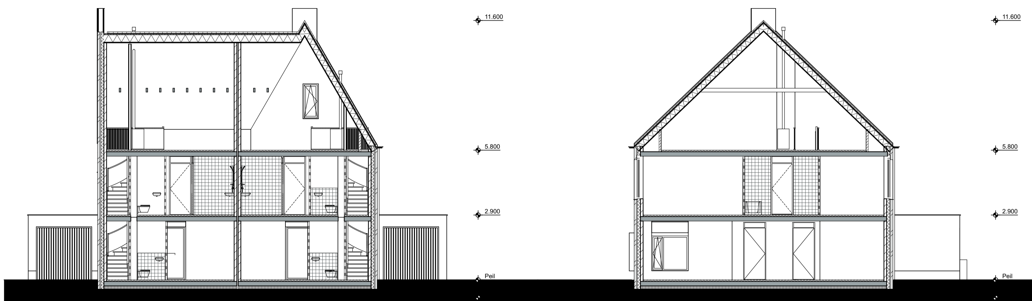
langsdoorsnede woning hoogte maatvoering in mm in plaats van cm
